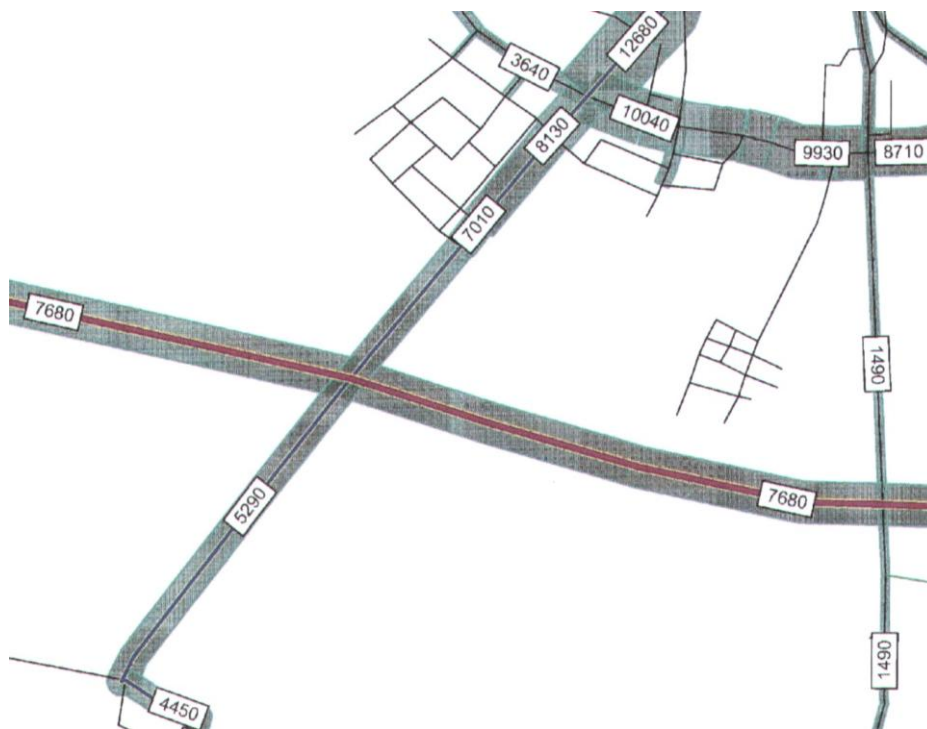
Ryc. 15. Kartogram średniodobowych natężeń ruchu kołowego w rejonie przecięcia DK 22 i DW 212 w Chojnicach, w roku 2015, w wariantcie bezinwestycyjnym 12 .
