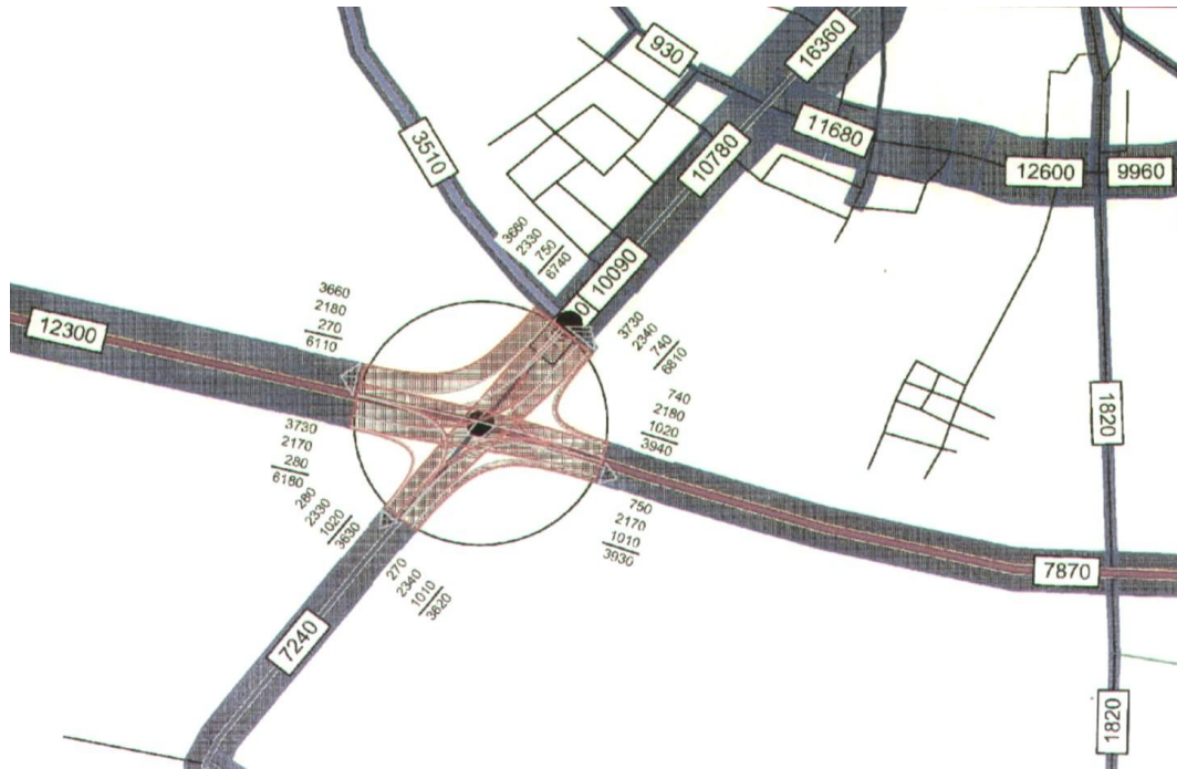
Ryc. 19. Kartogram średniodobowych natężeń ruchu kołowego w rejonie przecięcia DK 22 i DW 212 w Chojnicach, w roku 2035, w wariantcie bezinwestycyjnym 16 .
